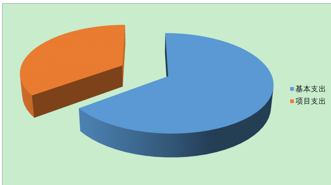
图2：支出预算图
